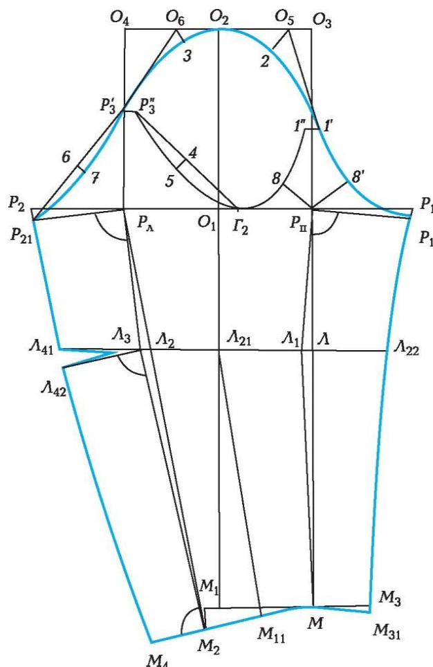
5.21. сурет Бір тігісті жеңнің сызбасы
