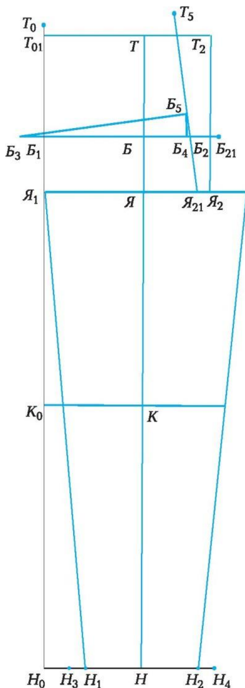
6.1. сурет. Ерлер шалбары құрылымы сызығының базистік кесте құрылымы
