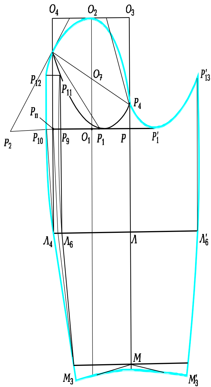
6.9 сурет. Біртігісті жеңнің құрылым сызбасы.
