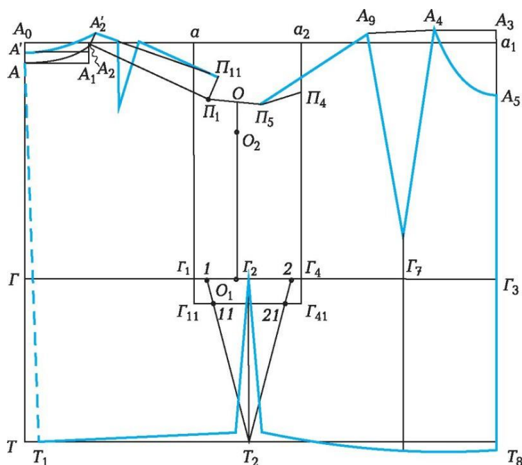
5.37 суреті. Жеңімен біртұтас пішілген бөлікше мен арқа бұйымының сызбасы
