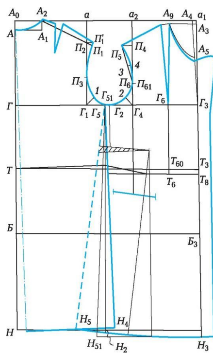
7.9. сурет Қыз балаға арналған тік сұлбалы маусымдық пәлліге негізінің сызбасы
