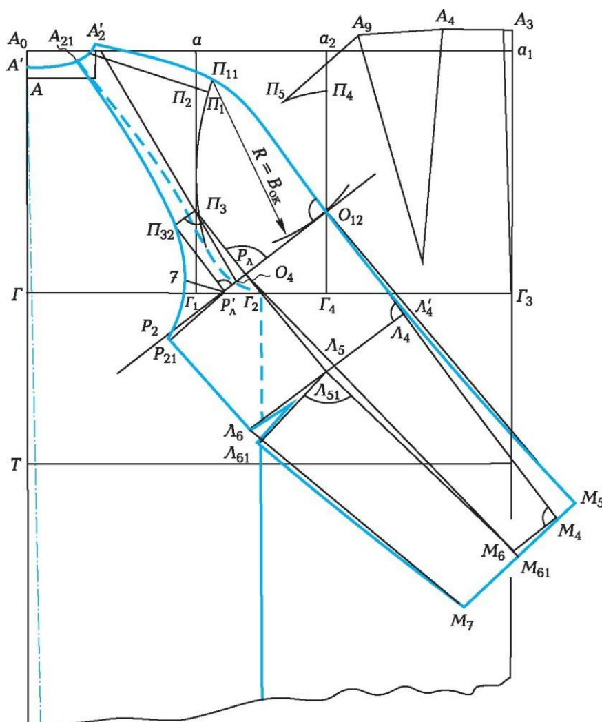
5.36. сурет. Реглан жеңінің артқы бөлігінің сызбасы
